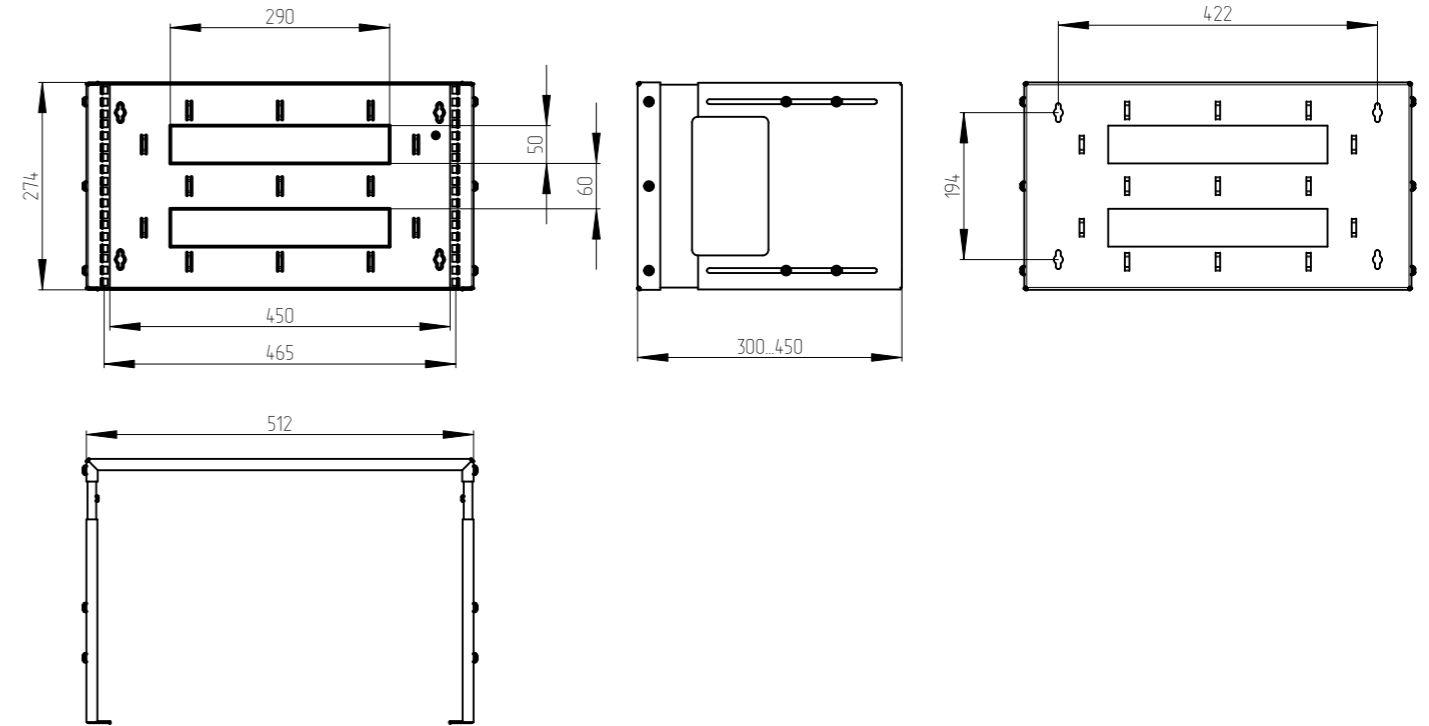
КНО-М-15U (Масштаб 1:10)
