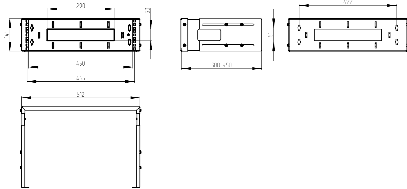
КНО-М-3U (Масштаб 1:10)
