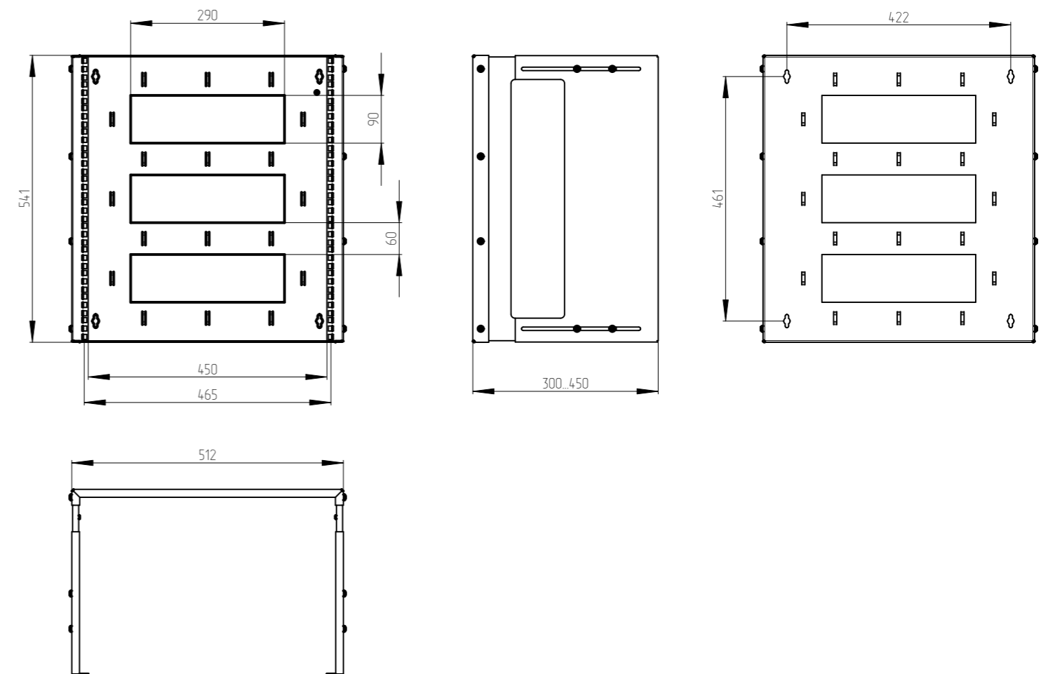
КНО-М-15U (Масштаб 1:10)
