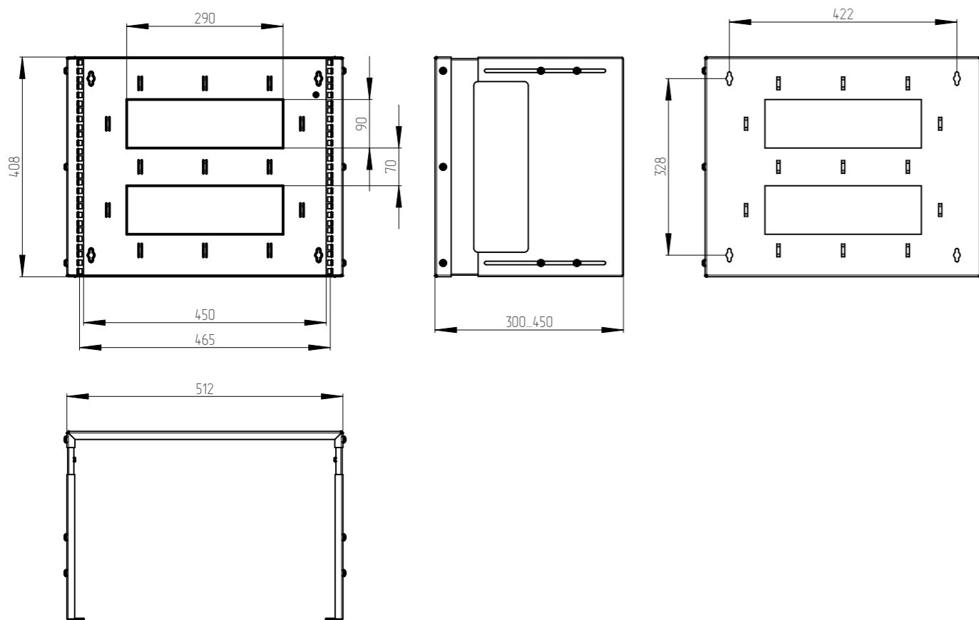
КНО-М-12U (Масштаб 1:10)
