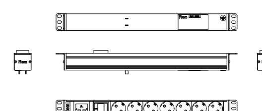
Блок розеточный R-16-7S-V-440
