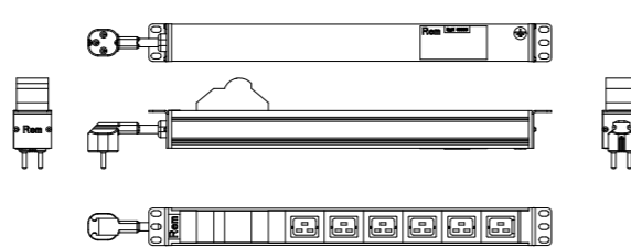
Блок розеточный R-16-6C19-A-440-3
